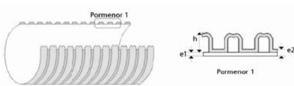
Tubos de pares doble
